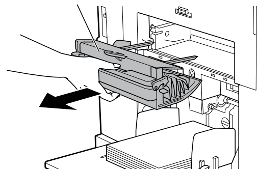
Griff des Masterauffangbehälters
